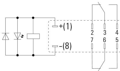
Вид на выводы снизу
