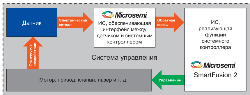
Рис. 3. Местоположение ИС LX3xx в АСУ
