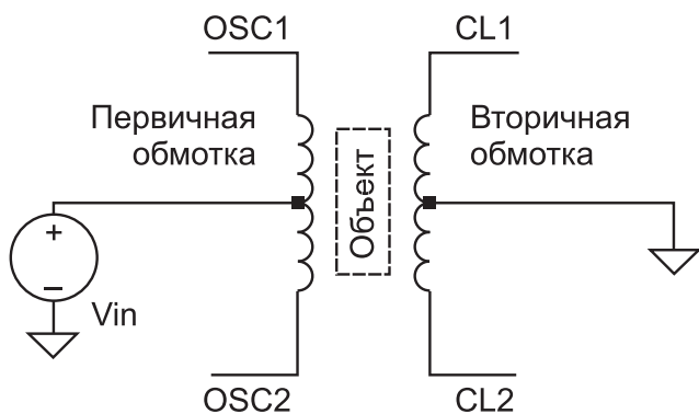
Рис. 1. Электрическая схема индуктивного датчика
